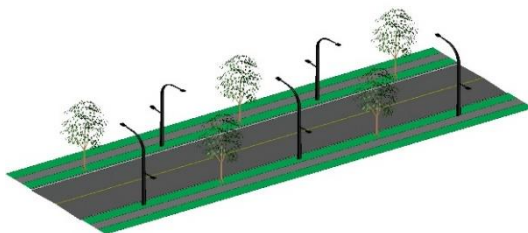
Figure 7 : Implantation en quinconce, dans un gabarit avec banquettes, avec des lampadaires combinés
