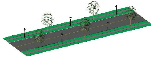
Figure 4 : Implantation en quinconce, dans un gabarit avec banquette, avec lampadaires décoratifs
