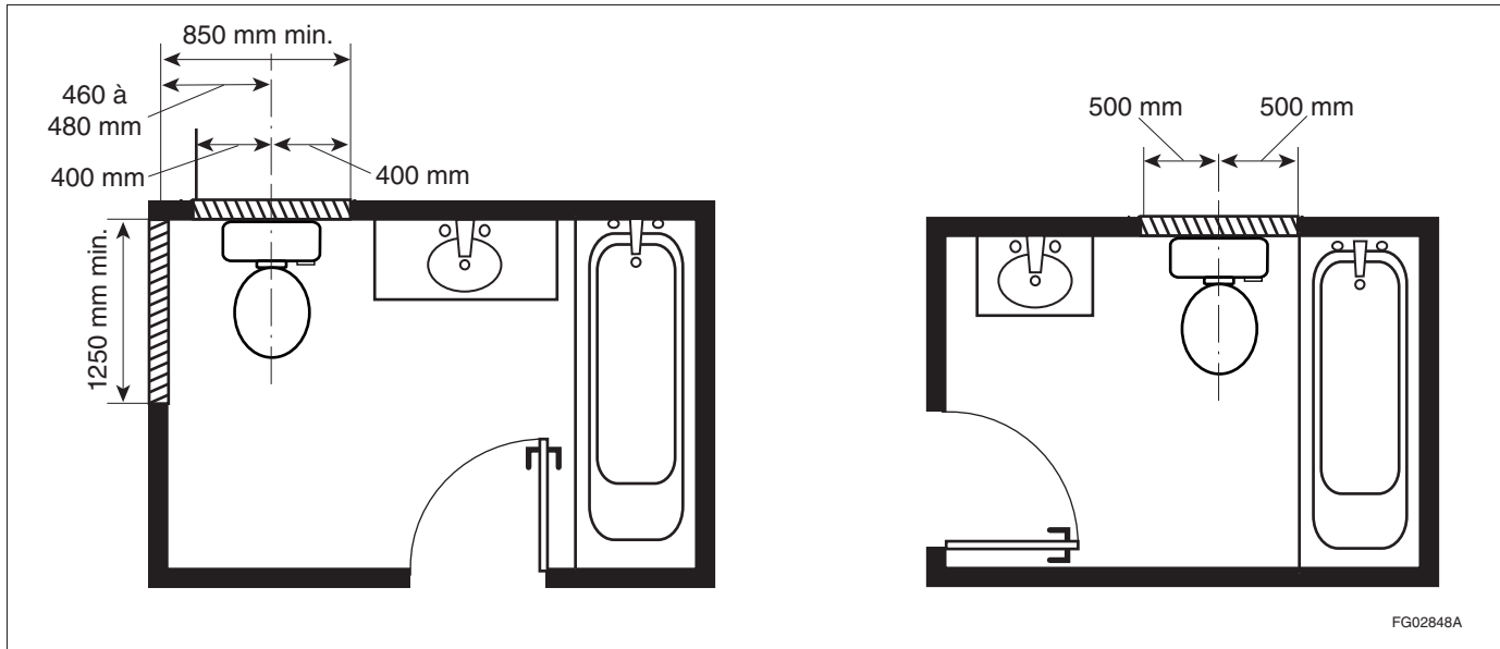
Figure A-3.8.4.5. 4) Fond de clouage pour l'installation des barres d'appui adjacentes au W.-C.
