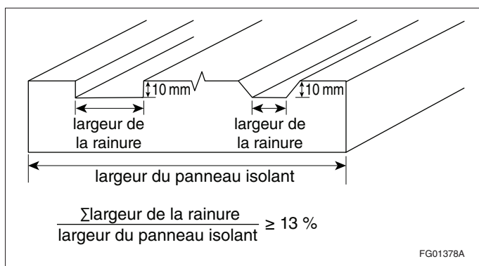
Figure A-9.27.13.1. 1) Cavity de drainage définie géométriquement
