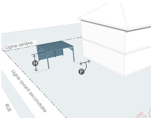
Figure 57. Distance minimale du bâtiment principal, retrait minimal par rapport au plan principal de la façade principale avant et hauteur maximale d'un pavillon de jardin
